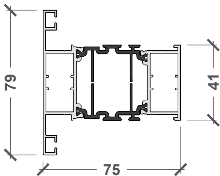
APX.DRT.079 79MM DOUBLE REBATE T
