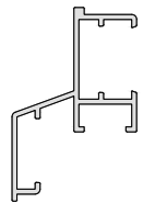
APX.ANC.101 VENT HOOD
