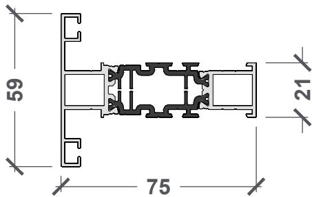
APX.DRT.059 59MM DOUBLE REBATE T
