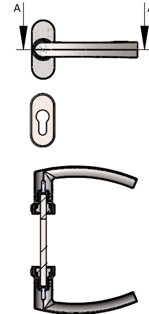
SECTION A-A SCALE 1 : 5
