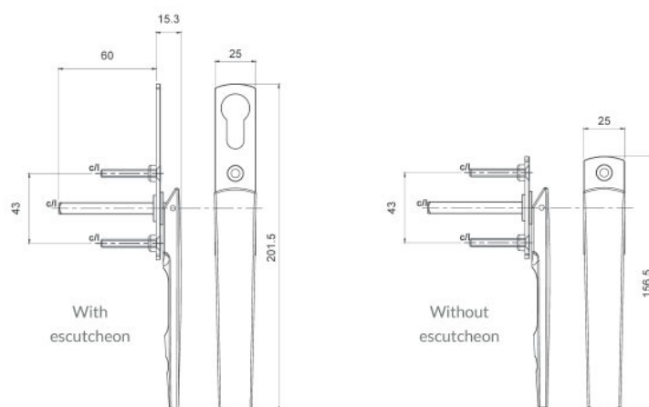
Shootbolt Handle
